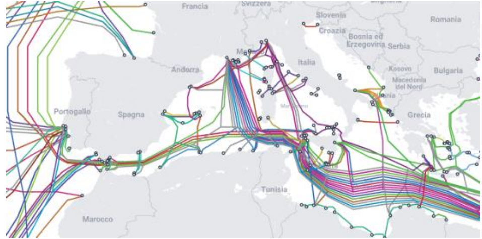
Analisi raggiungibilità fibra ottica Terrestri e sottomarini
